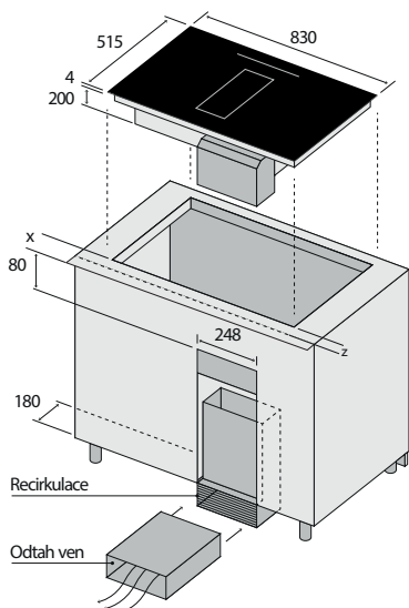
Instalace v rovině s deskou
