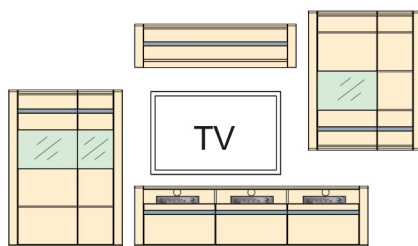
Art. č.: Kombi 04 pre každú medzeru je pripočítaných 100 mm S V H 3452 1987 504 pozostáva z: Typ 04 1 ks Typ 32 1 ks Typ 22 1 ks Typ 41 1 ks 580-0369/022
