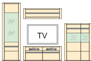
Art. č.: Kombi 01 pre každú medzeru je pripočítaných 100 mm S V H 3153 2048 504 pozostáva z: Typ 01 1 ks Typ 31 1 ks Typ 04 1 ks Typ 41 1 ks 580-0369/019
