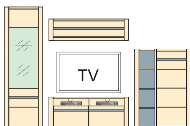
Art. č.: Kombi 02 pre každú medzeru je pripočítaných 100 mm S V H 3153 2048 504 pozostáva z: Typ 01 1 ks Typ 31 1 ks Typ 06 1 ks Typ 41 1 ks 580-0369/020
