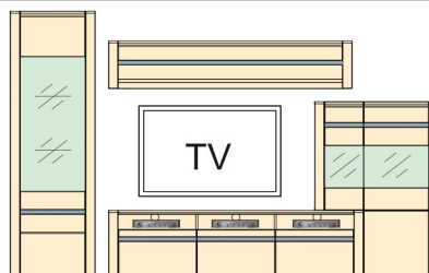
Art. č.: Kombi 110 pre každú medzeru je pripočítaných 100 mm S V H 3278 2048 504 pozostáva z: Typ 01 1 ks Typ 32 1 ks Typ 12 1 ks Typ 09 1 ks Typ 43 1 ks 580-0369/028
